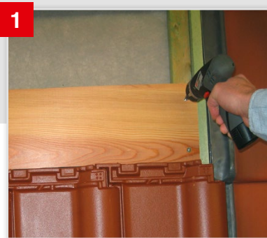
1 Holzbohle in Stärke der Traglatte (ca. 160 mm breit) direkt oberhalb der Dachziegel in die Tragkonstruktion befestigen.
