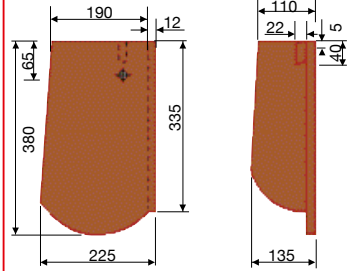
1 1/4 Ortgang rechts 22,5/38 Rundschnitt
