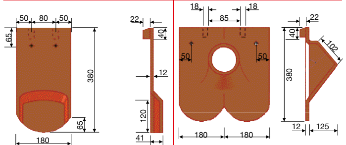
Biberlüfter 18/38 Rund-/Geradschnitt
