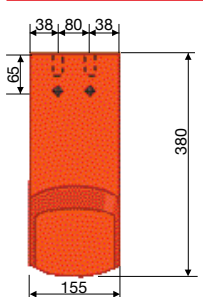
Biberlüfter 15,5/38 Berliner Biber
