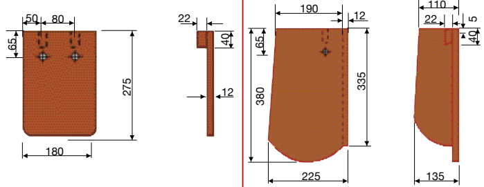
Traufbiber 18/27,5 Rundschnitt
