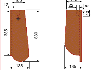
3/4 Ortgang links 13,5/38 Rundschnitt
