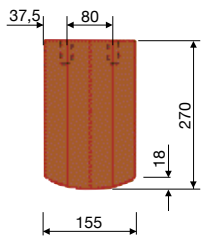
Flächenbiber 15,5/38 Berliner Biber
