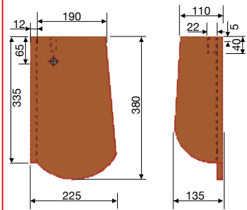
1 1/4 Ortgang links 22,5/38 Rundschnitt
