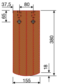
Flächenbiber 15,5/38 Berliner Biber
