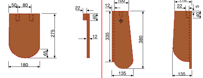
Firstbiber 18/27,5 Rundschnitt
