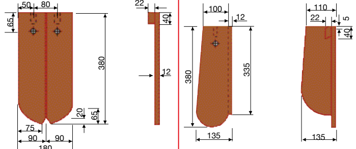
1/2 Biber, teilbar 18/38 Rundschnitt
