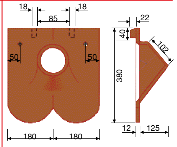
Durchgangsbiber 36/38 Rund-/Geradschnitt
