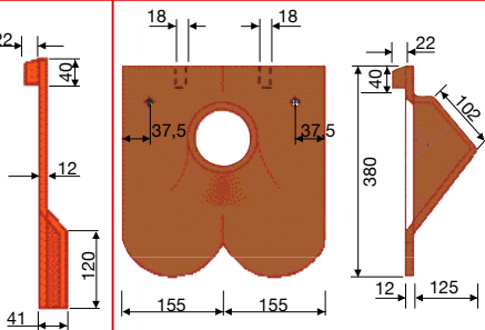
Durchgangsbiber 31/38 Berliner Biber
